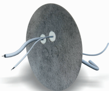
hySeal Multi mit 4 Kabeldurchgängen von Ø 3-15 mm. Eine für alle Kabel mit Manschettenknopf-Verschlussstechnik
