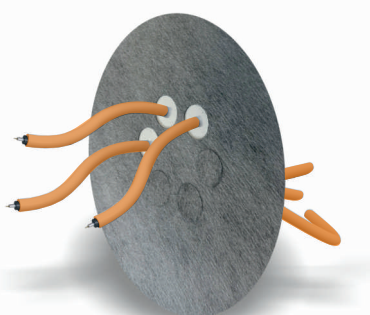
hySeal LAN - mit 6 geöffneten Kabeldurchgängen. Eine für alle LAN-Kabel mit Manschettenknopf-Verschlussstechnik
