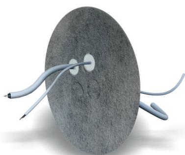
hySeal Multi mit 4 Kabeldurchgängen von Ø 3-15 mm. Eine für alle Kabel mit Klebepatch Verschlusstechnik
